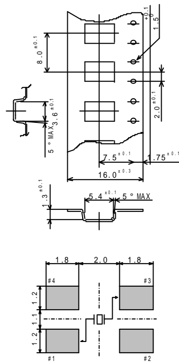
ランドパターン参考図 (TOP VIEW)
